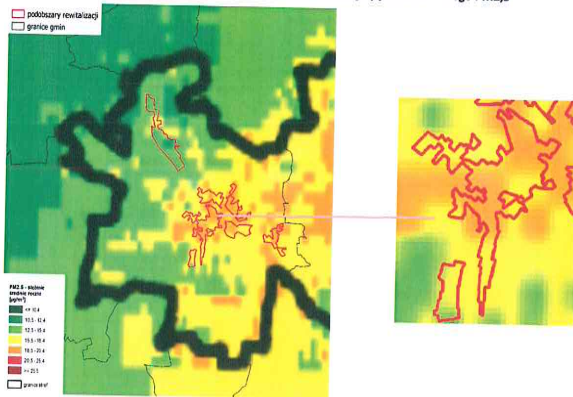
Mapa 45. Rozkład przestrzenny wartości stężenia średniorocznego pyłu zawieszonego PM 2,5
