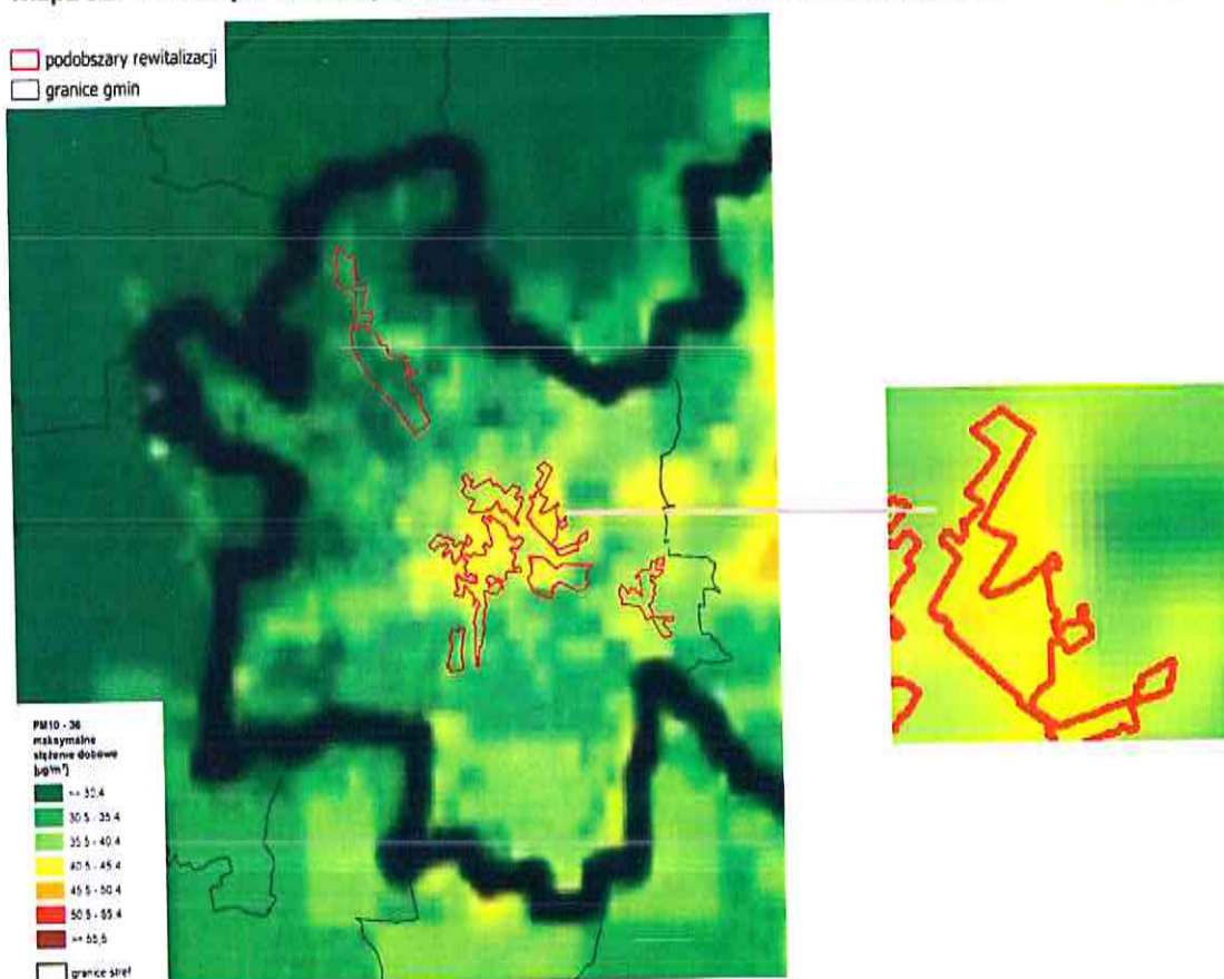
Mapa 51. Rozkład przestrzenny 36 maksymalnej wartości stężenia 24-godzinnego pyłu zawieszonego PM10
