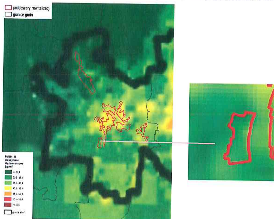
Mapa 31. Rozkład przestrzenny 36 maksymalnej wartości stężenia 24-godzinnego pyłu zawieszonego PM10
