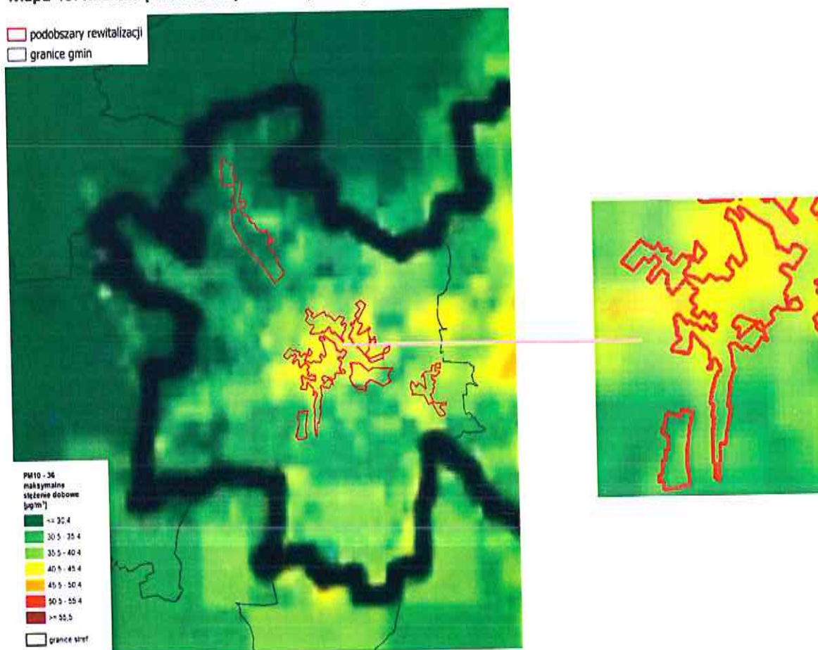
Mapa 46. Rozkład przestrzenny 36 maksymalnej wartości stężenia 24-godzinnego pyłu zawieszonego PM10
